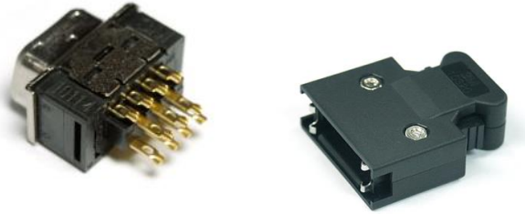
[그림 3-4 External IO 커넥터 (MDR10114-300PE)]
