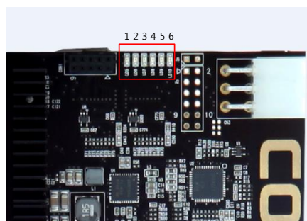
[그림 3-7 보드 동작상태 확인 LED]
