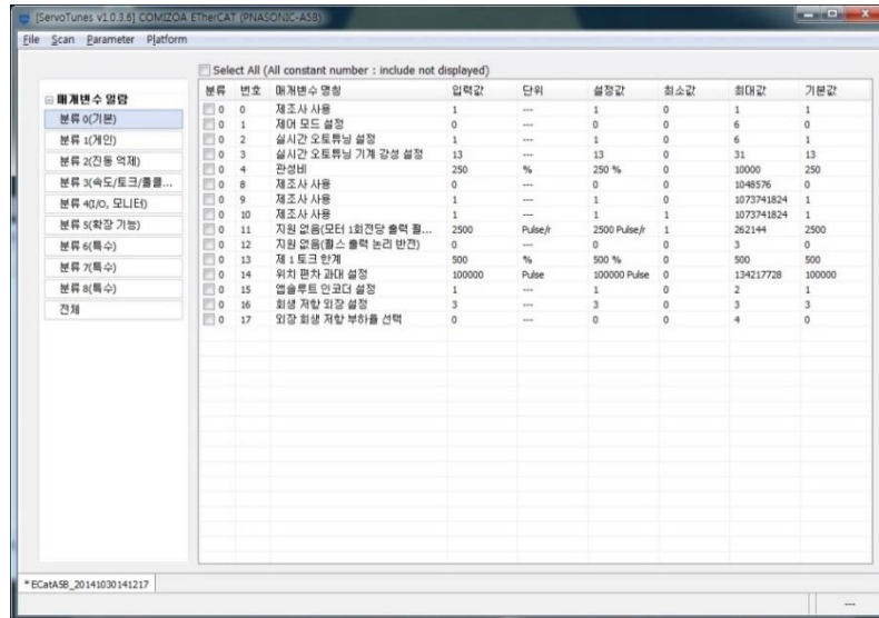
[그림 1-7] ServoTunes
