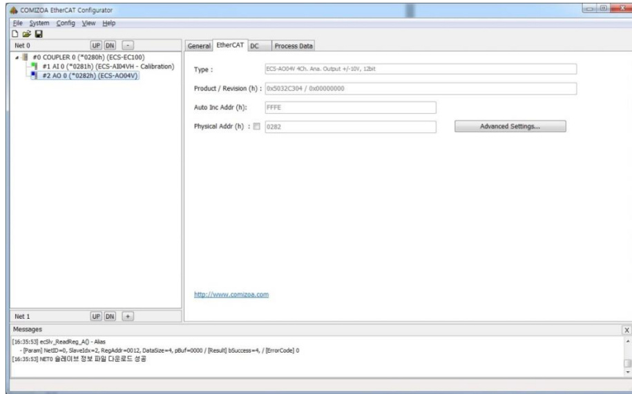
[그림 1-5] COMI-Configurator
