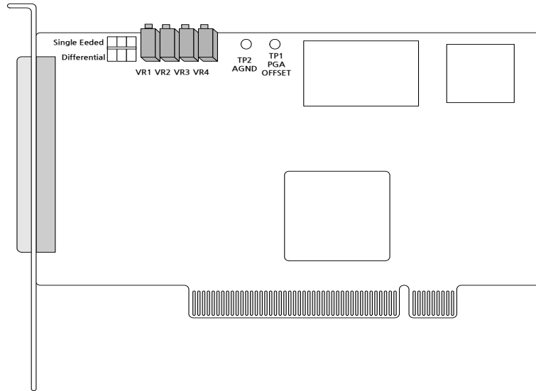
[그림 A-3] COMI-SD201 Calibration 용 가변 저항의 위치
