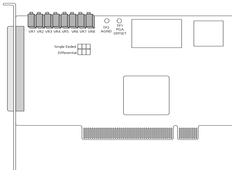
[그림 A-1] COMI-SD101/103 Calibration 용 가변 저항의 위치
