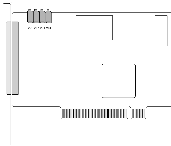
[그림 A-2] COMI-CP101 Calibration 용 가변 저항의 위치
