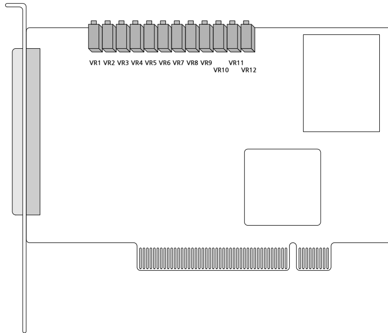
[그림 A-5] COMI-CP301 Calibration 용 가변 저항의 위치
