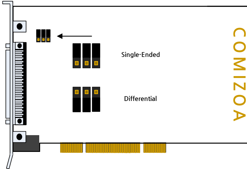
[그림 1-6] COMI-SD Series AD Mode Jumper
