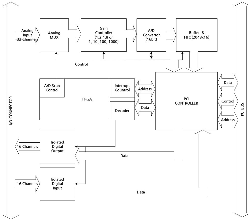
[그림 1-2] COMI-SD203 Hardware 개념도
