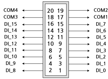
[그림 1-4] COMI-SD203 커넥터 P1 핀 배열
