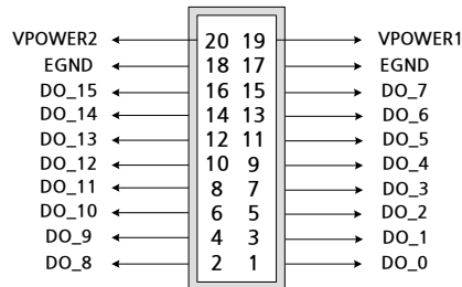
[그림 1-5] COMI-SD203 커넥터 P2 핀 배열
