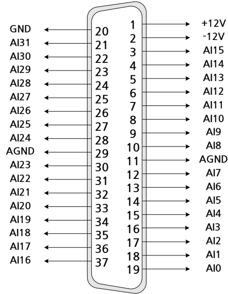
[그림 1-3] COMI-SD203 커넥터 핀 배열
